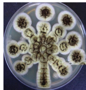
Aspergillus
